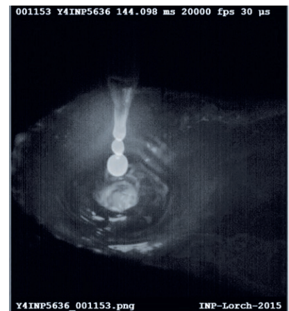
Der Primärtropfen geht ins Schmelzbad über und die Sekundärtropfen lösen sich.
