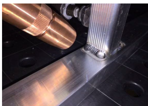
Aluminium Geländerrahmen
